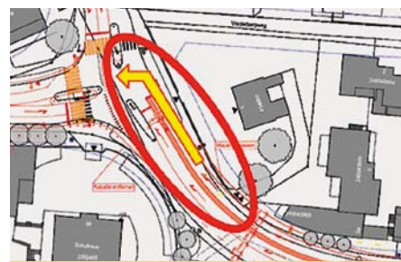
Neue Busspur in die Bahnhofstrasse
